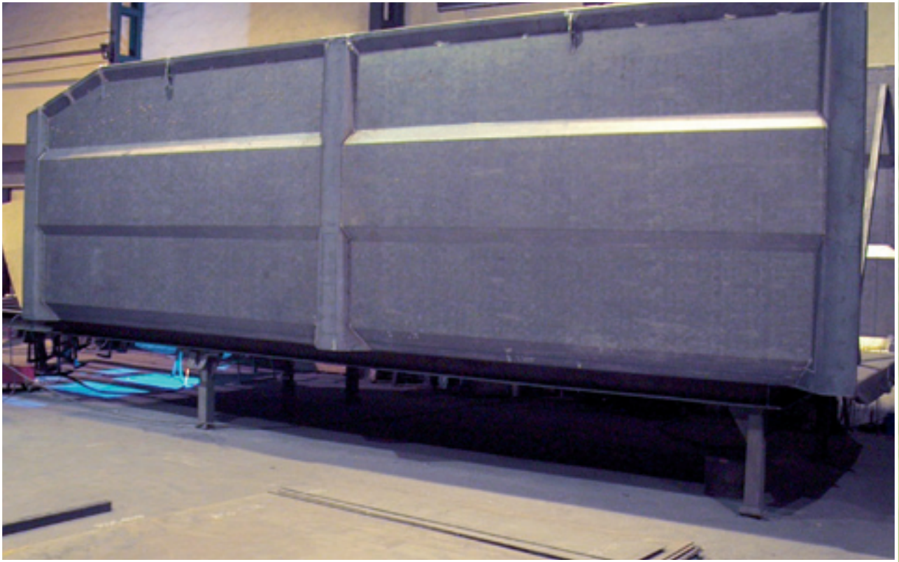
Montaje de caja chatarrera en chapa especial 6 mm. "ROC-450".
