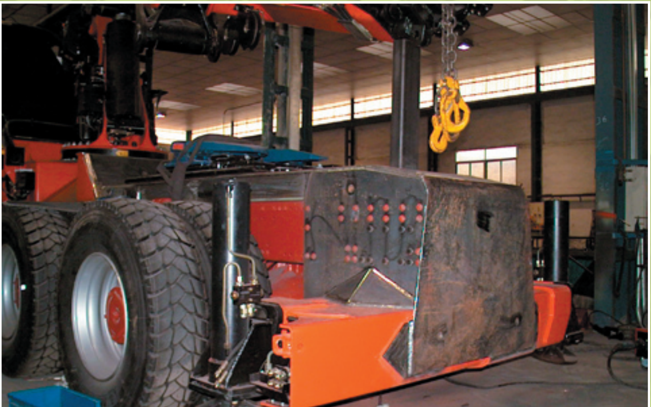
Montaje de Estabilizadores traseros de grúas de gran tonelaje.
