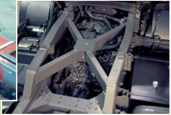
Refuerzos antitorsión en zona de grúa mediante cruz de San Andrés.
